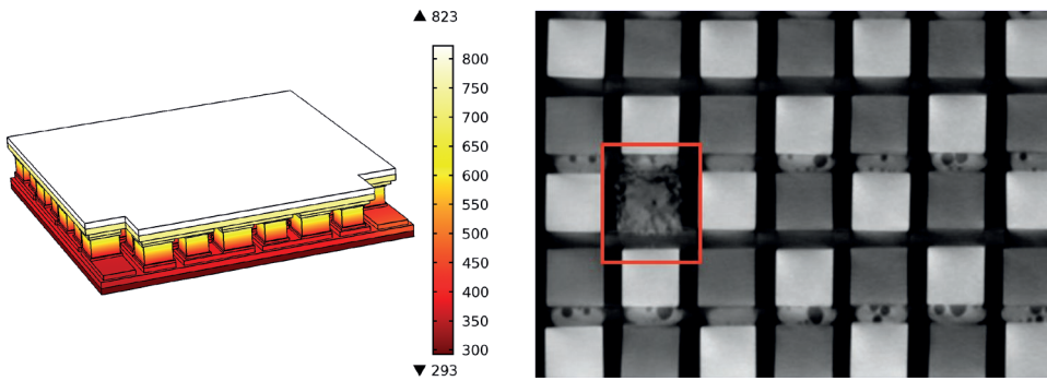
FEM-Simulation der Temperaturverteilung in einem Peltier-Modul mit einer festen Heiß- und Kaltseiten-Temperatur von 800 und 25 °C. Thermo-elektrische Effekte sind in der zugrundeliegenden Simulation ebenfalls berücksichtigt.
